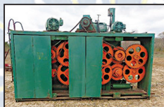
Nicholson A5 22" Ring (2) Available
