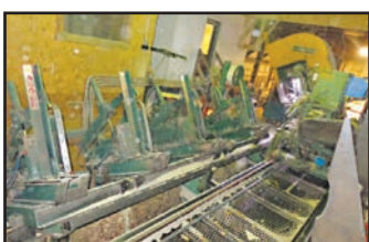
Sanborn Mini Max w/4 H.B. Cleereman Carriage
