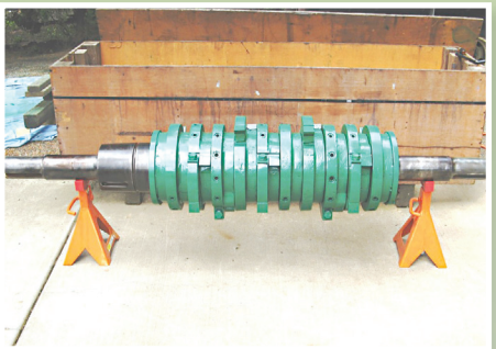
42HD-ER Hog Rotor, 10365
